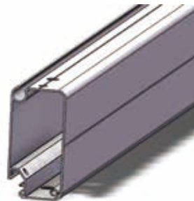
名称：中横梁 材质：铝合金 规格：80*40*1.4mm Name: Middle crossbeam Material: Aluminum alloy Specifications: 80*40*1.4mm
