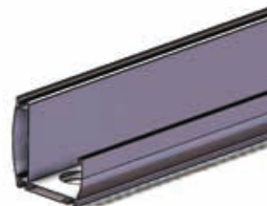
名称：水槽 材质：铝合金 规格：157.7*154*1.6mm Name: Gutter Material: Aluminum alloy Specifications: 157.7*154*1.6mm
